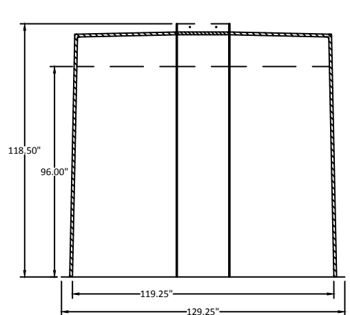
RIGHT ELEV.
