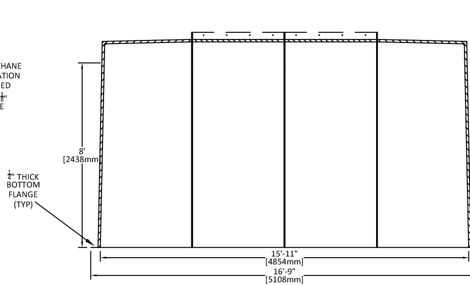
RIGHT ELEV.
