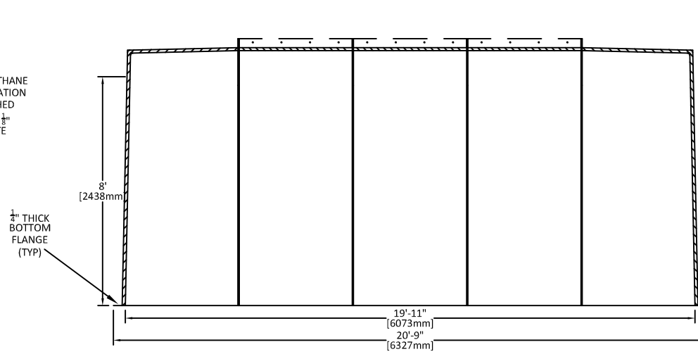
RIGHT ELEV.
