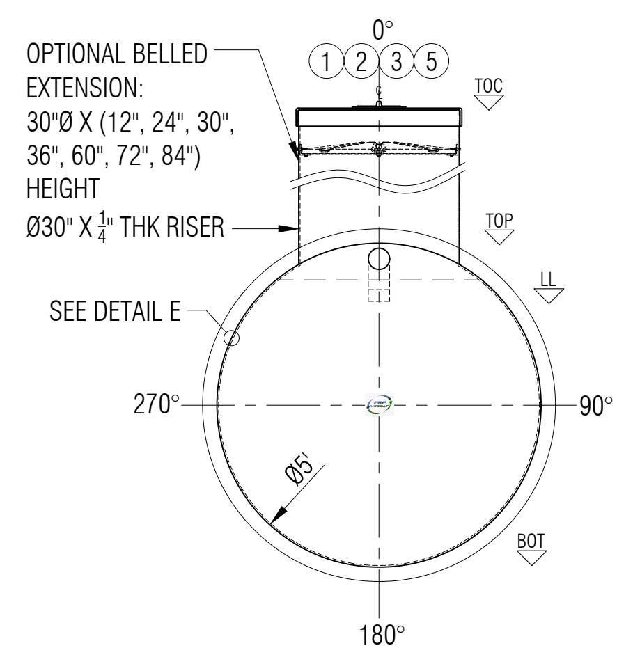
ELEVATION B
